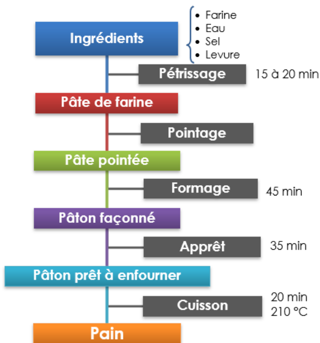
Figure 3. Diagramme simplifié de la fabrication du pain.
