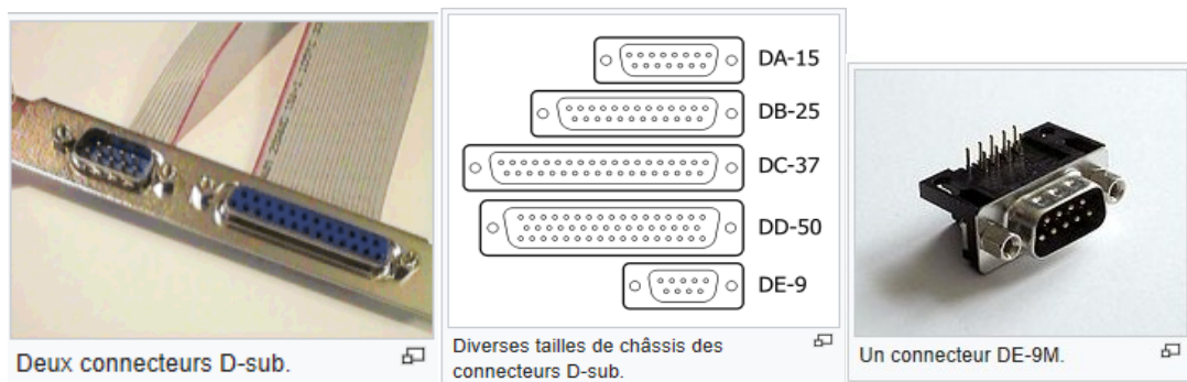
Figure 4.2 Les différents connecteurs Sub-D
